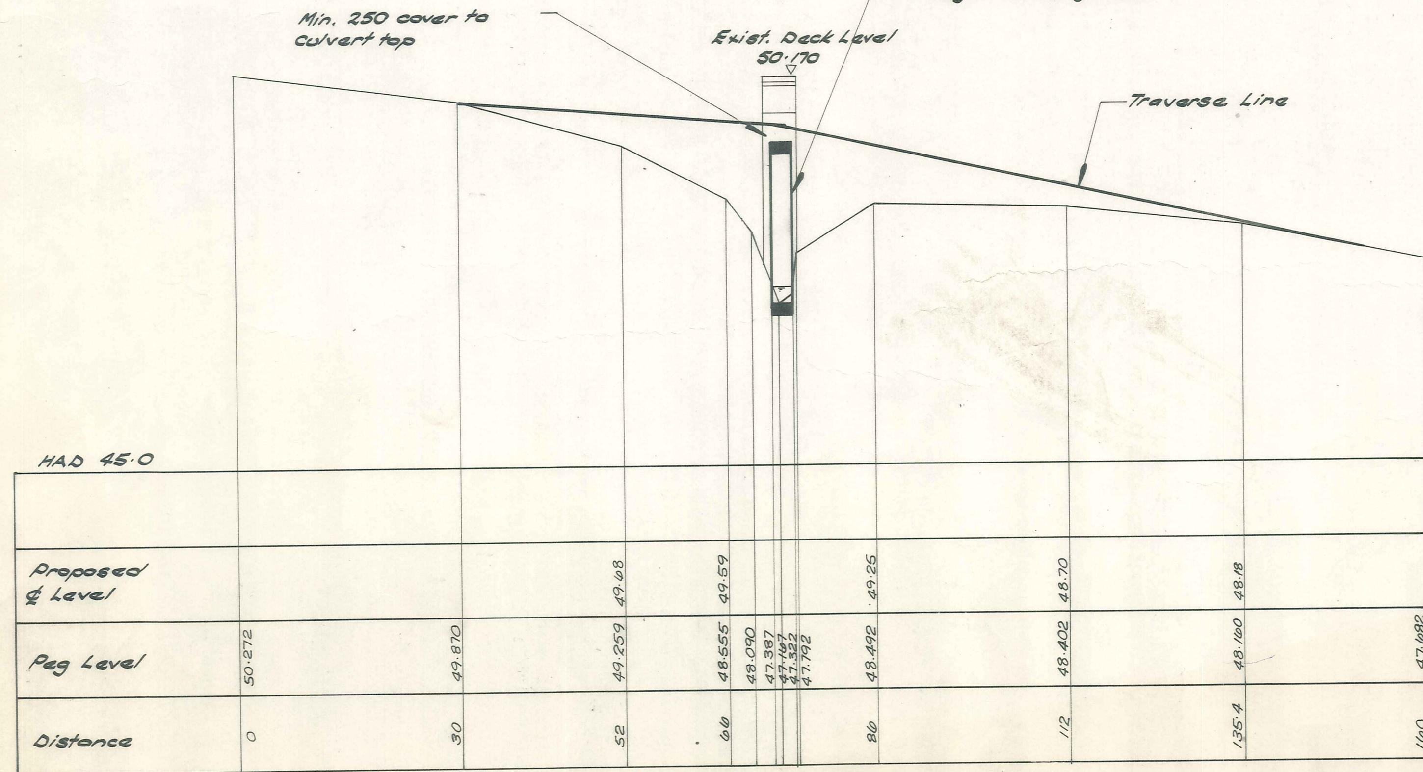
LONGITUDINAL SECTION Scale; Horiz. 1:500 Vert. 1:50
